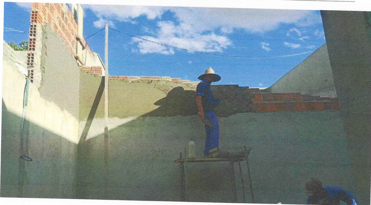
Foto 19 - MASSA ÚNICA, PARA RECEBIMENTO DE PINTURA, EM ARGAMASSA TRAÇO 1:2:8, PREPARO MECÂNICO COM BETONEIRA 400L, APLICADA MANUALMENTE EM FACES INTERNAS DE PAREDES, ESPESSURA DE 10MM, COM EXECUÇÃO DE TALISCAS. AF_06/2014
