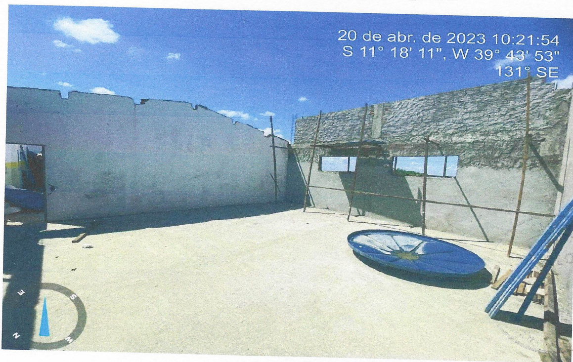
Foto 18 - CHAPISCO APLICADO EM ALVENARIAS E ESTRUTURAS DE CONCRETO INTERNAS, COM COLHER DE PEDREIRO. ARGAMASSA TRAÇO 1:3 COM PREPARO EM BETONEIRA 400L. AF_06/2014
