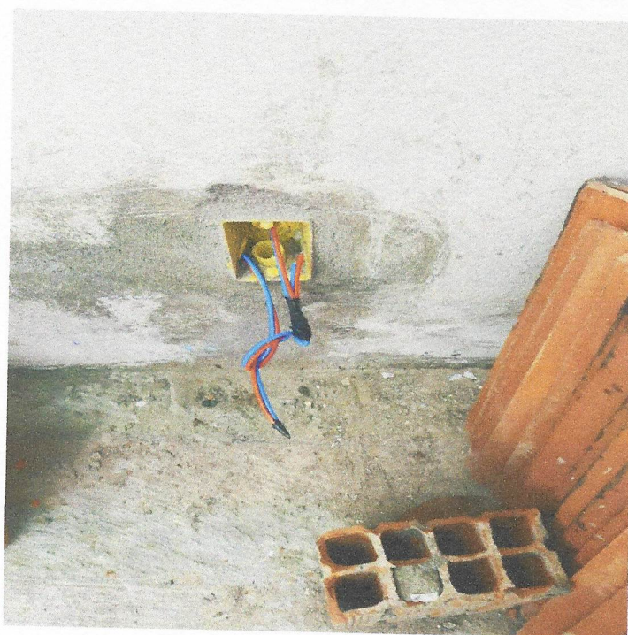
Foto 16 - CABO DE COBRE FLEXÍVEL ISOLADO, 2,5 MM 2 , ANTI-CHAMA 450/750 V, PARA CIRCUITOS TERMINAIS - FORNECIMENTO E INSTALAÇÃO. AF_12/2015
