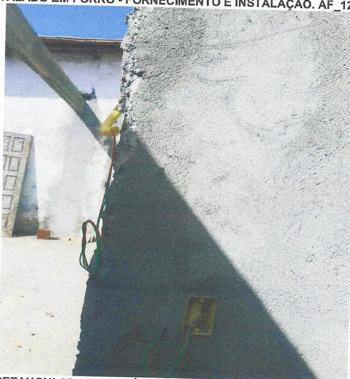
Foto 14 - CAIXA RETANGULAR 4" X 2" MÉDIA (1,30 M DO PISO), PVC, INSTALADA EM PAREDE - FORNECIMENTO E INSTALAÇÃO. AF_12/2015
